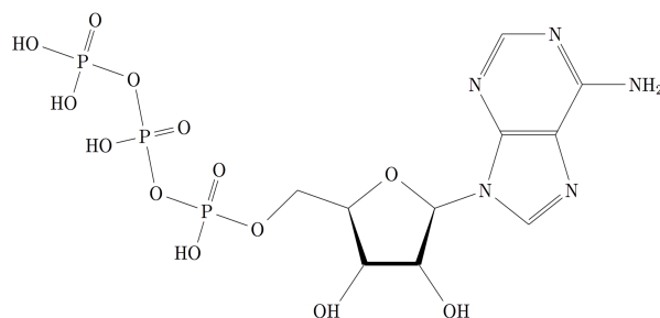
FIGURE 3 – molecule en formule developpée : graphe non orienté et annoté
