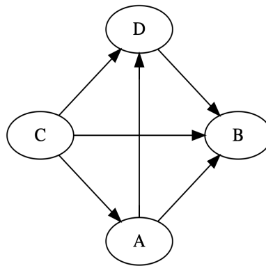
FIGURE 4 – graphe orienté du tournoi
